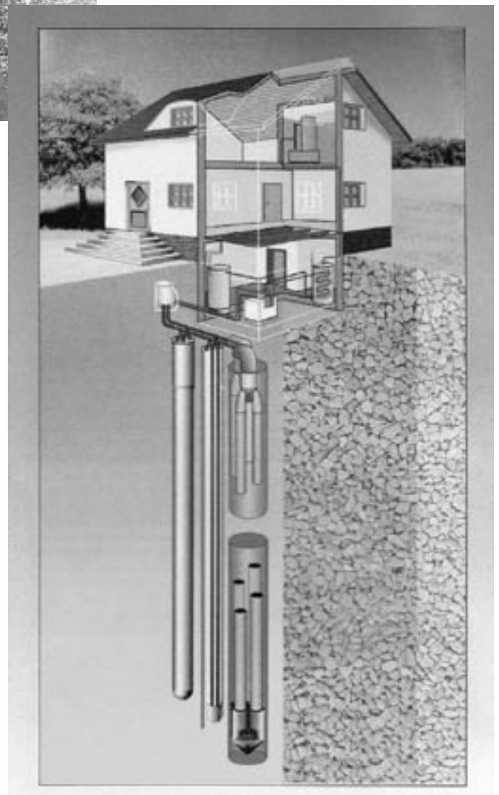
Funktion der Erdwärmesonden
